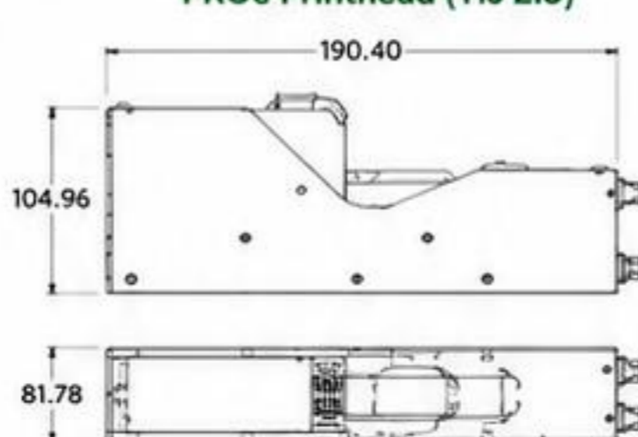
PROe Printhead (TIJ 2.5)
