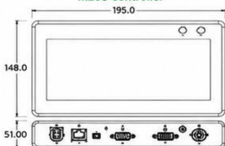
M20e Controller
